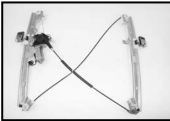
19. ACI Part No 82123 07-99 Chevrolet, Cadillac, & GMC
